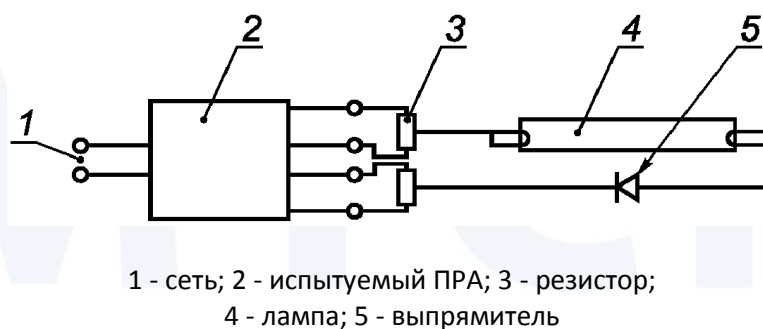
Рисунок С.1. Схема проверки выпрямительного эффекта (только для бесстартерных емкостных ПРА)
