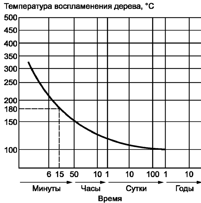
Рисунок 27. Температура воспламенения дерева в функции времени
