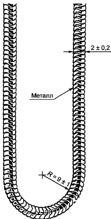
Рисунок 29. Цепь для испытаний
