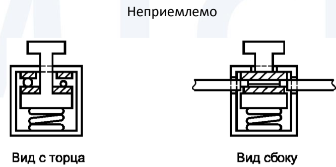
Рисунок 18. Примеры безвинтовых контактных зажимов пружинного типа
