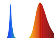
Спектрограмма излучения
