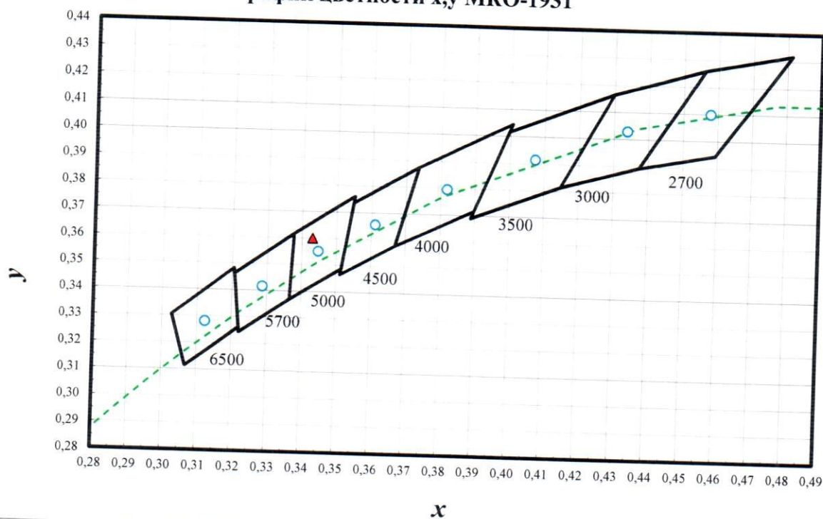
График цветности x, y МКО-1931
