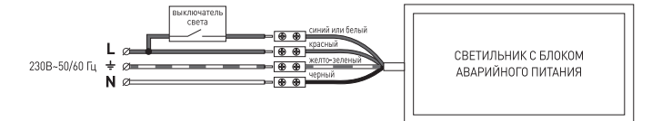
Նկ.1 Լամպը 230Վ-ցանցին միացնելու սխեմա
