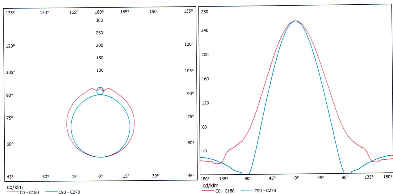
Рисунок 3 – График КСС образца в декартовых координатах
