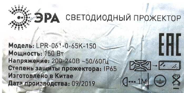
Маркировка прожектора
