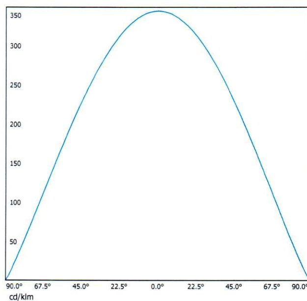
Рисунок 3 – График КСС образца в декартовых координатах
