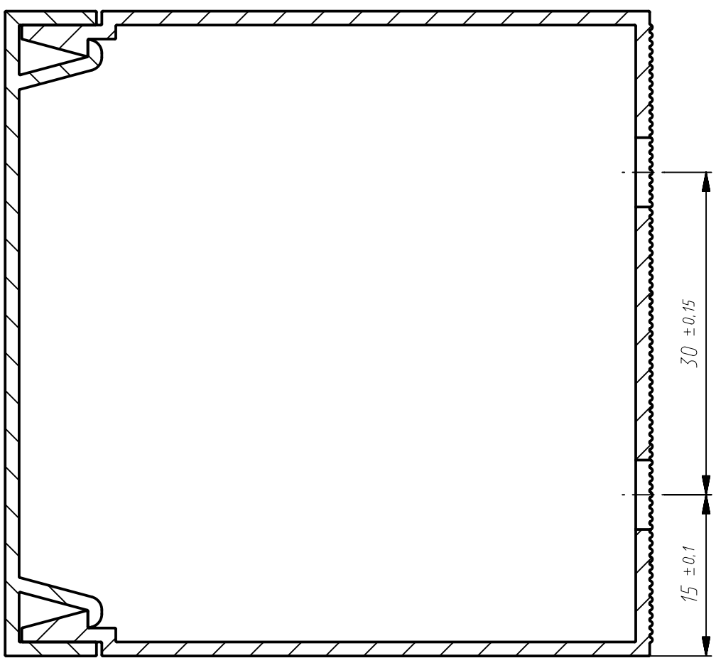
A-A (2:1)
