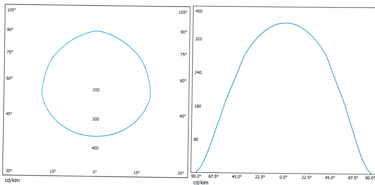
Рисунок 2 – График КСС образца в полярных координатах
