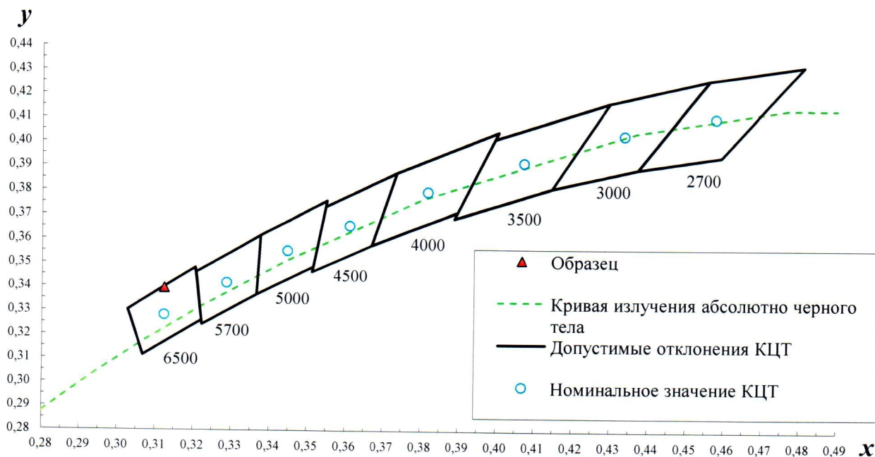
Рисунок 1 – Положение образца на графике цветностей МКО 1931 г.
