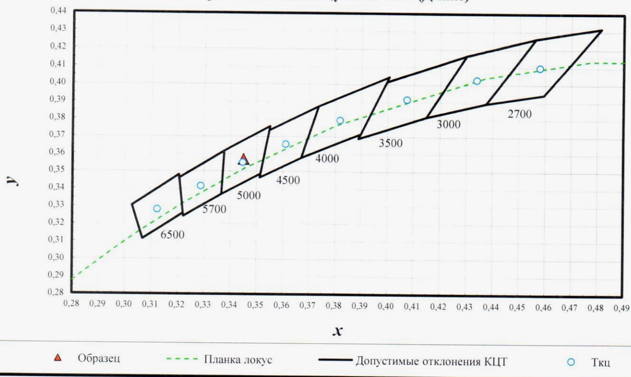
Диаграмма цветности x, y МКО-1931 (Дмакс)
