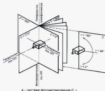
а - система фотометрирования C, \gamma
