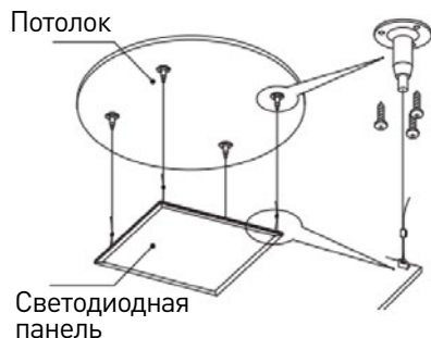
Крепление SPL-FIX1 Б0019797
