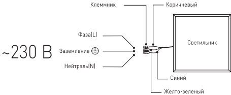
Рис.1. 230В шамчыракты токо туташтыруу схемасы
