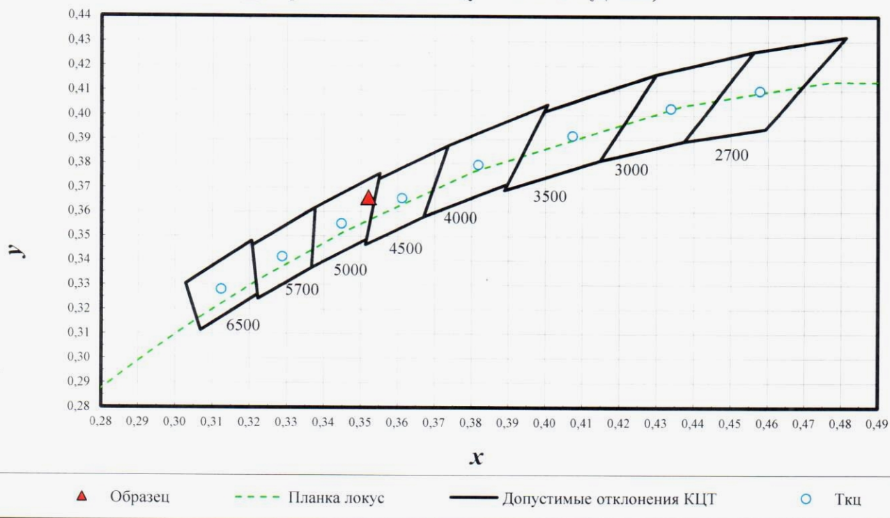
Диаграмма цветности x, y МКО-1931 (Дмакс)
