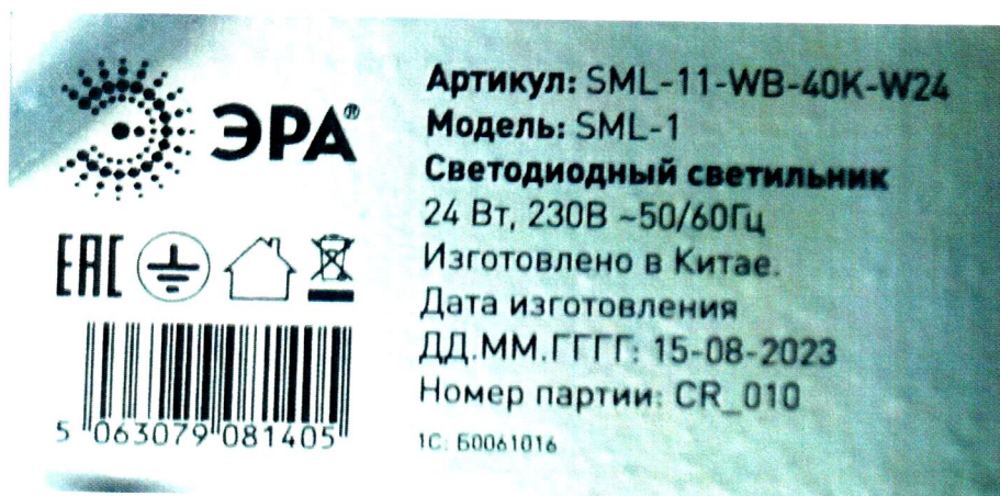
Рисунок А.1 – Фотография маркировки образца
