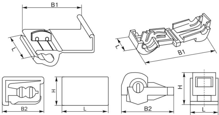
Рисунок 1 Габаритные и установочные размеры ответвителей
