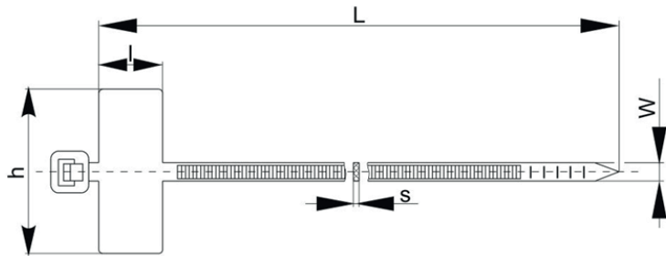
б) Габаритные размеры хомутов NO-225-320 Рисунок 1 Габаритные размеры хомута
