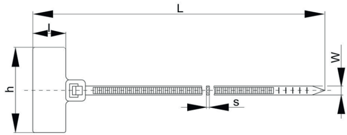
а) Габаритные размеры хомутов NO-225-318, NO-225-319
