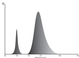
СӘУЛЕЛЕНУ СПЕКТРГРАММАСЫ
