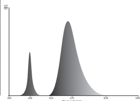
СНУРДАНУУНУН СПЕКТРОГРАММАСЫ
