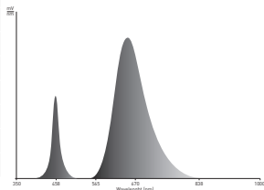
СПЕКТРОГРАММА ИЗЛУЧЕНИЯ
