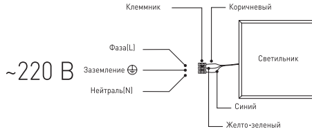
Рис.1. 220В шамчыракты токою туташтыруу схемасы
